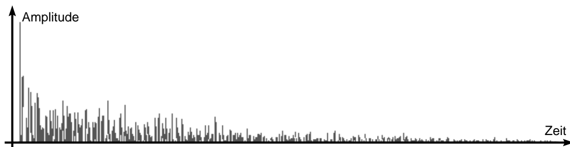
Abbildung 1: Impulsantwort eines Raumes, bestimmt durch dessen Architektur
